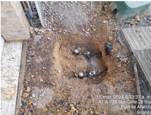
ANTES: Acometidas a nueva tubería de PVC – Zanja abierta
